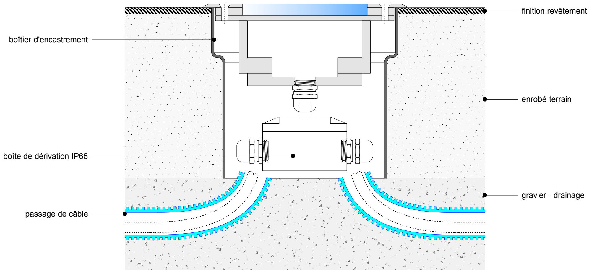
Détail pour une connexion IP dans la boîte de dérivation
