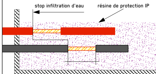
Détail pour une connexion IP dans la boîte de dérivation
